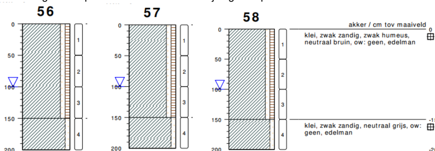
Afbeelding 3: Boorprofielen raai meest westelijke gedempte sloot
