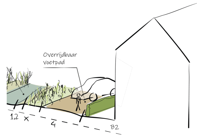
Principeprofiel overrijdbaar voetpad
