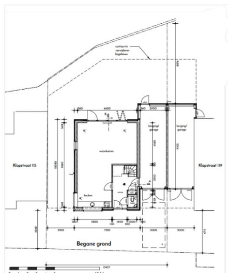
Figuur 2.10 Indelingsschets van het bovenaanzicht van de begane grond van het nieuw te bouwen woonhuis (bron: Jan Jansen Bouwkundig Adviseurs).
