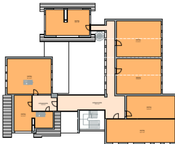
eerste verdieping
